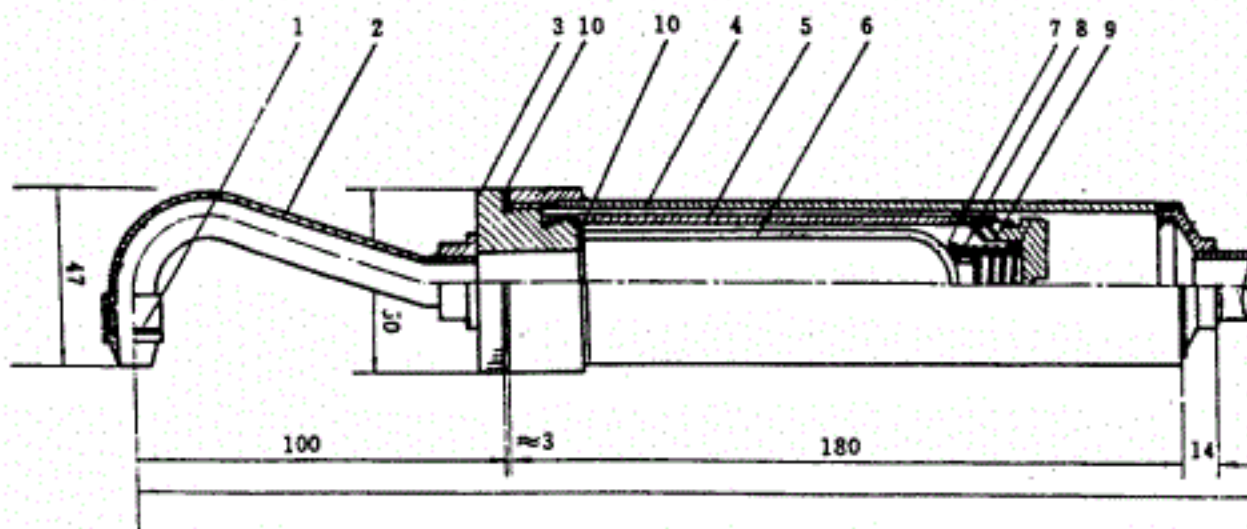
图 21 刚玉滤筒采样管
