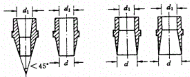
图22 采样嘴
