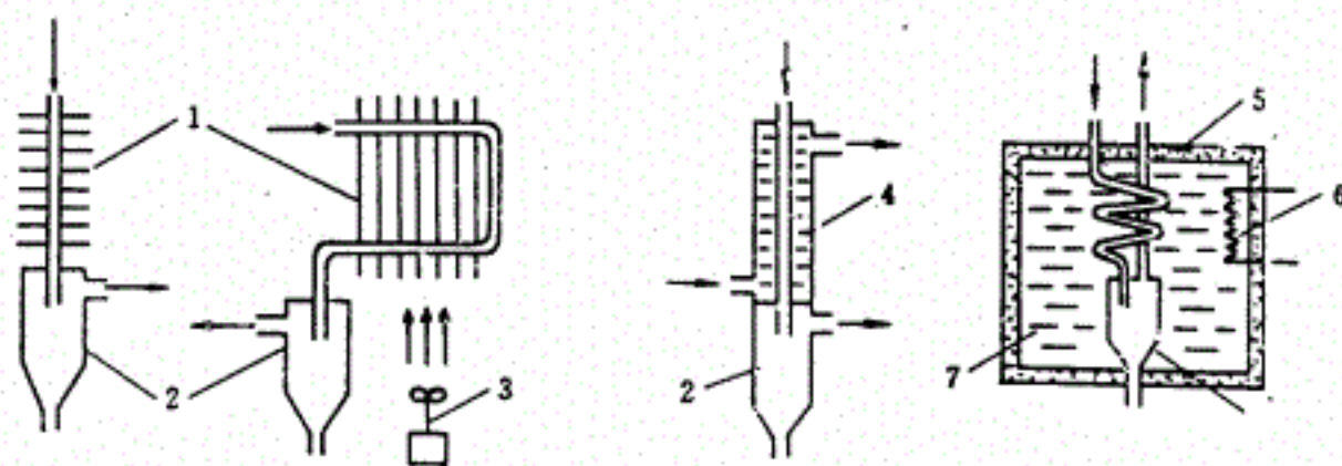
图 33 常用的几种除湿器
