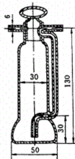
图 14 雪菲尔德吸湿管
