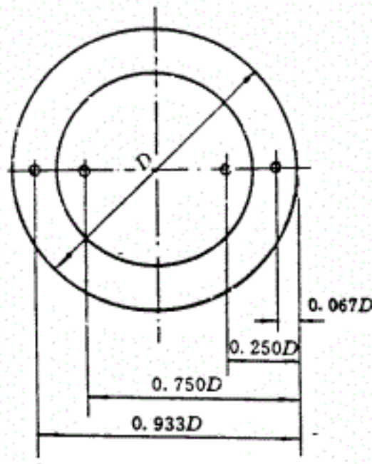
图 9 采样点距烟道内壁距离
