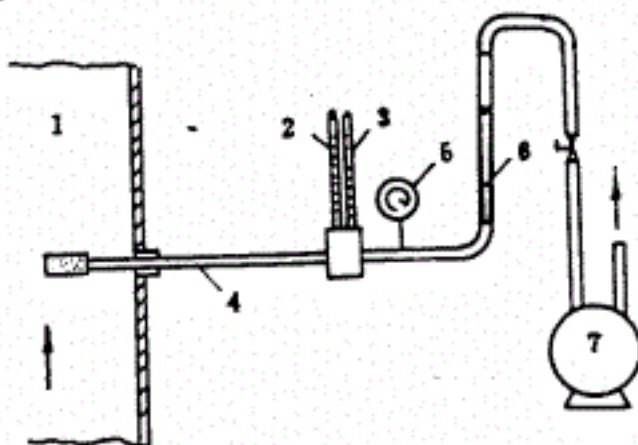
图 11 干湿球法测定排气水分含量装置
