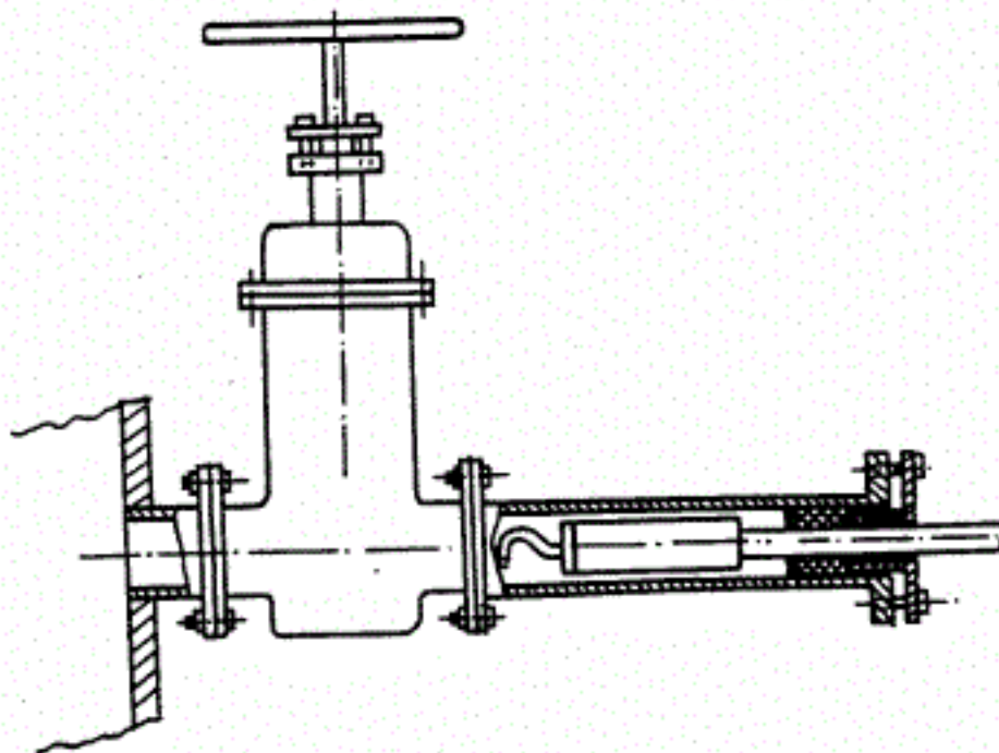
图 4 带有闸板阀的密封采样孔
