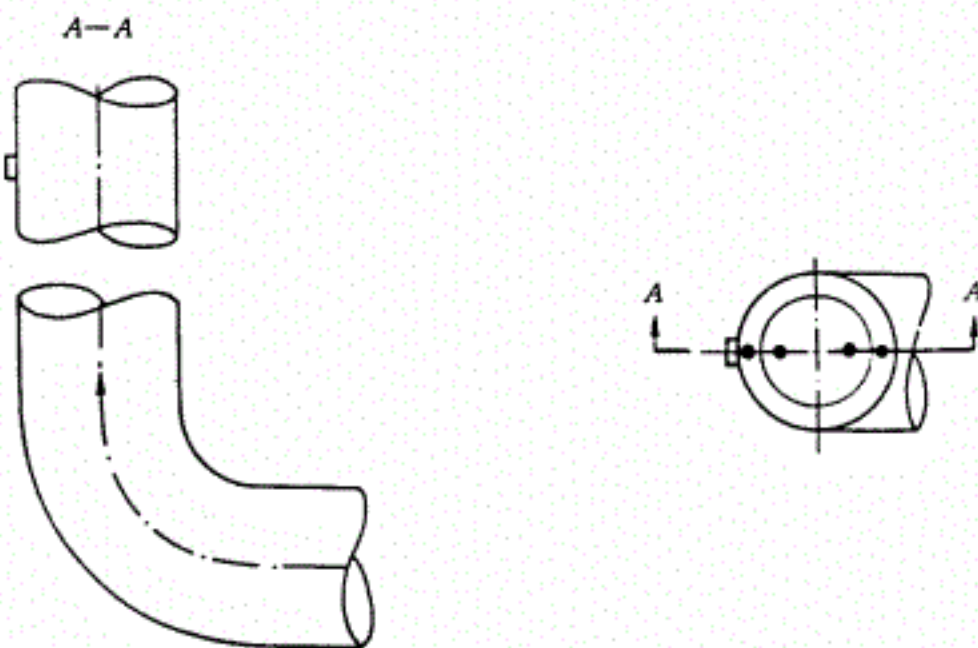
图8 圆形烟道弯头后的测点
