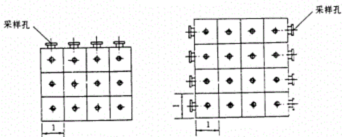
图7 正方形断面的测定点
