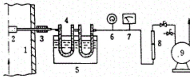
图 12 重量法测定排气水分含量装置
