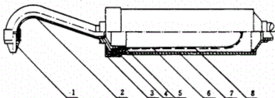
图 20 玻璃纤维滤筒采样管
