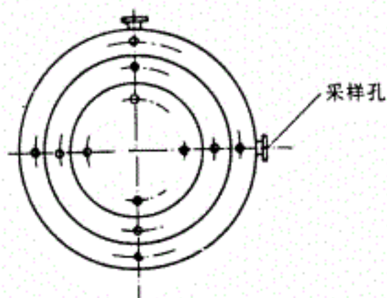
图5 圆形断面的测定点
