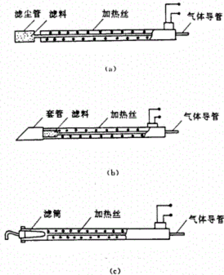
图 32 几种加热式采样管
