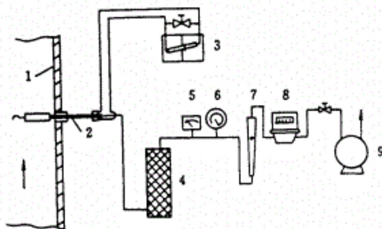
图 26 静压平衡法固体颗粒物采样装置
