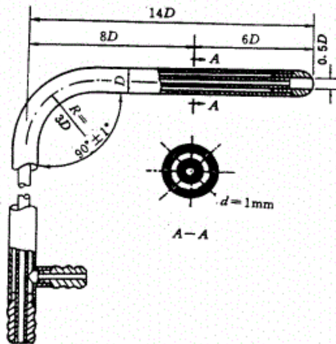
图 16 标准型皮托管
