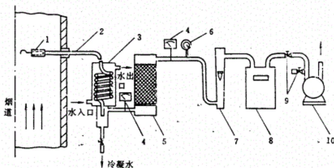
图 10 冷凝法测定排气水分含量装置
