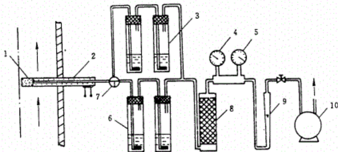
图 28 烟气采样系统
