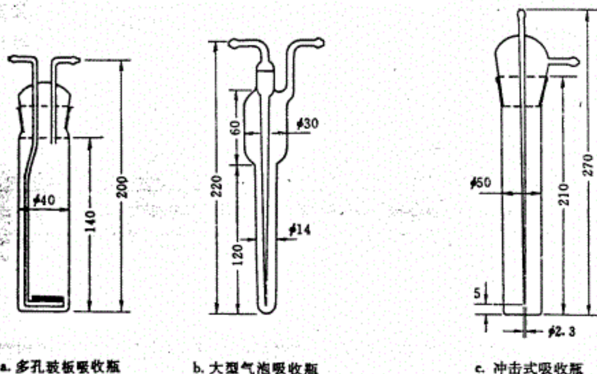
图 34 常用的几种吸收瓶
