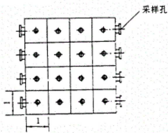
图7 正方形断面的测定点
