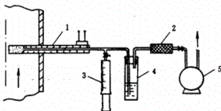
图 30 注射器采样系统
