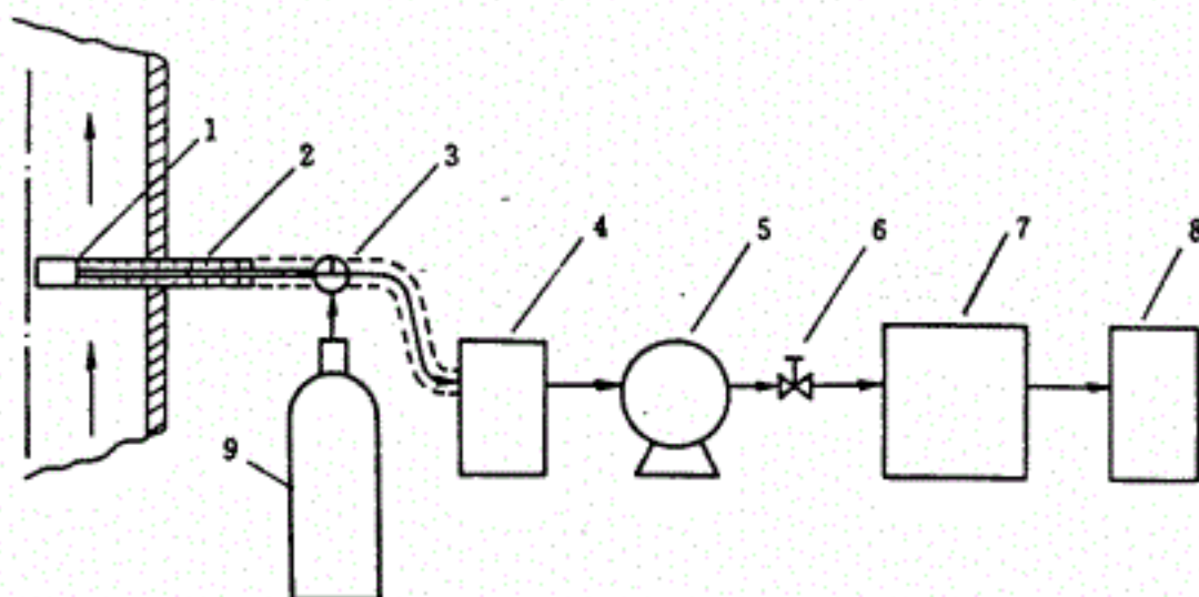
图 31 仪器测试法采样系统
