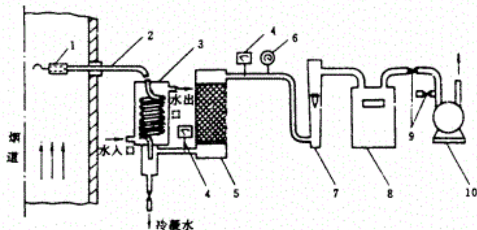
图 19 普通型采样管法颗粒物采样装置
