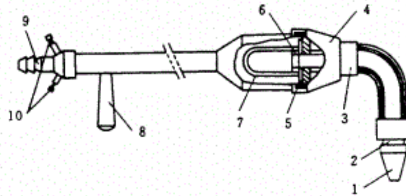
图 27 静压平衡采样管结构
