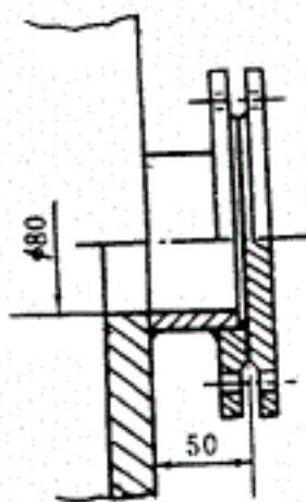
图 1 带有盖板的采样孔 (单位: mm)
