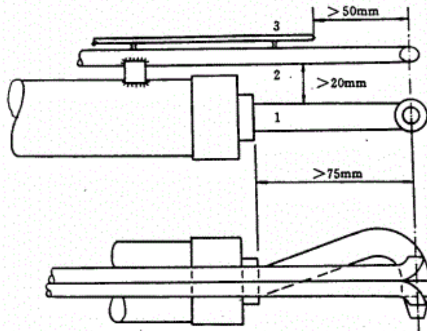
图 24 组合采样管相对位置要求
