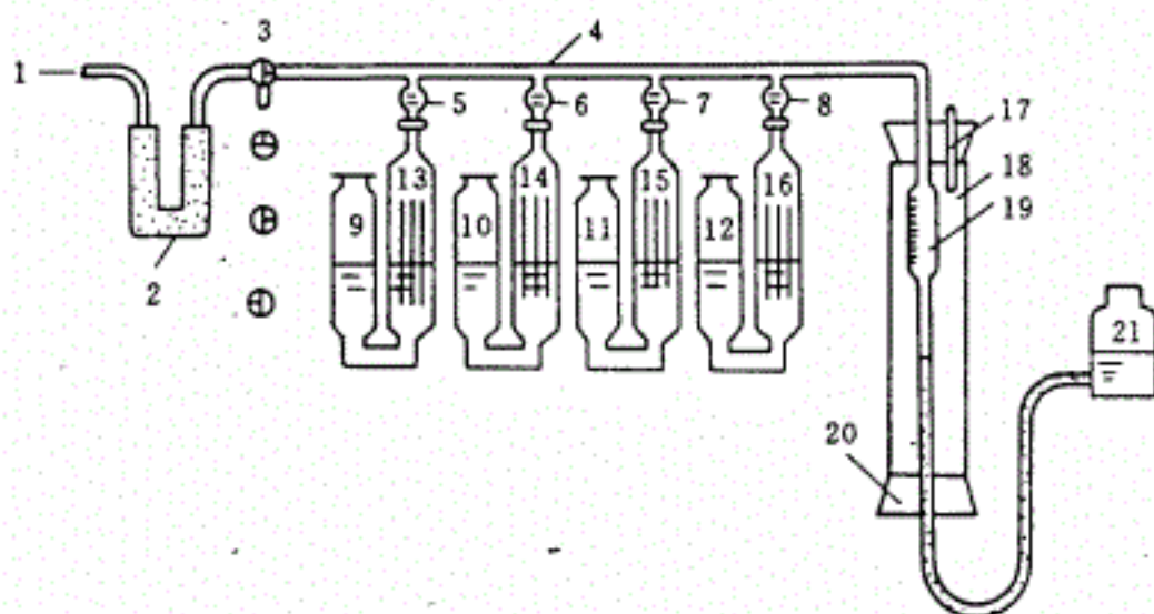
图 15 奥氏气体分析仪
