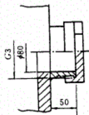
图 3 带有管帽的采样孔 (单位: mm)
