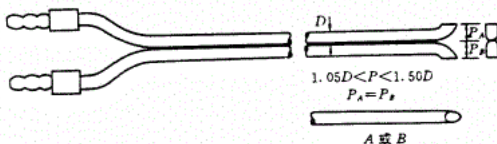
图 17 S 型皮托管
