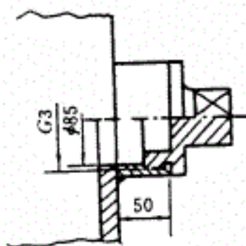
图 2 带有管堵的采样孔 (单位: mm)
