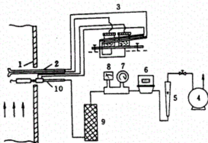
图 25 动压平衡法固体颗粒物采样装置
