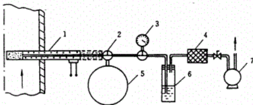
图 29 真空瓶采样系统
