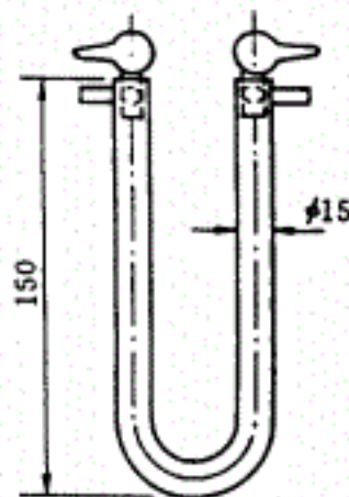
图 13 U 形吸湿管
