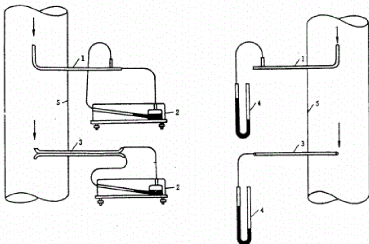
图 18 动压及静压的测定装置
